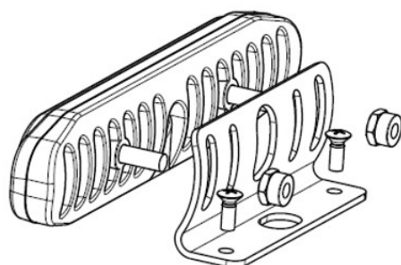
Uchycení za pomoci uchycovací destičky tvaru „L“
