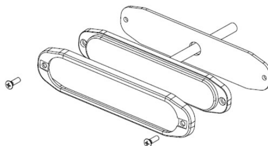
Povrchové uchycení pomocí uchycovací destičky „U“
