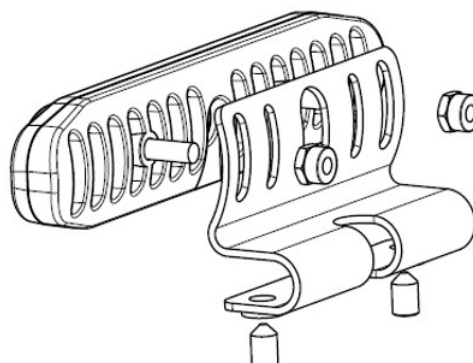
Povrchové uchycení pomocí uchycovací destičky „U“
