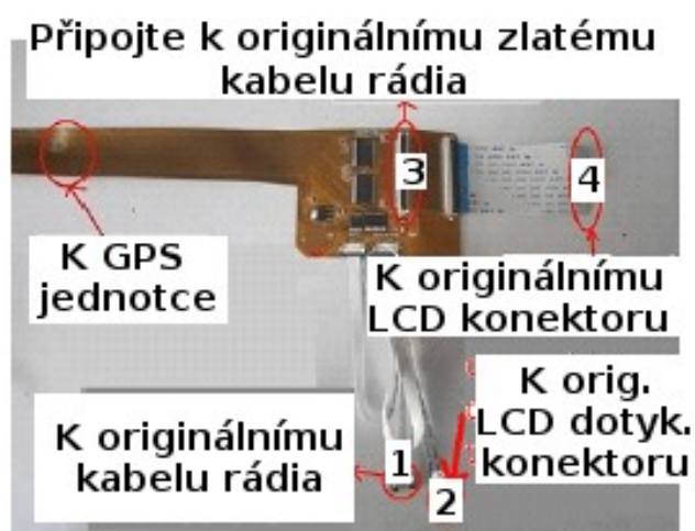
Zlatý FPC kabel adaptéru
